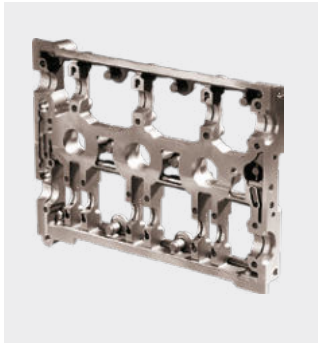
Leiterrahmen für Nockenwellenlagergehäuse
